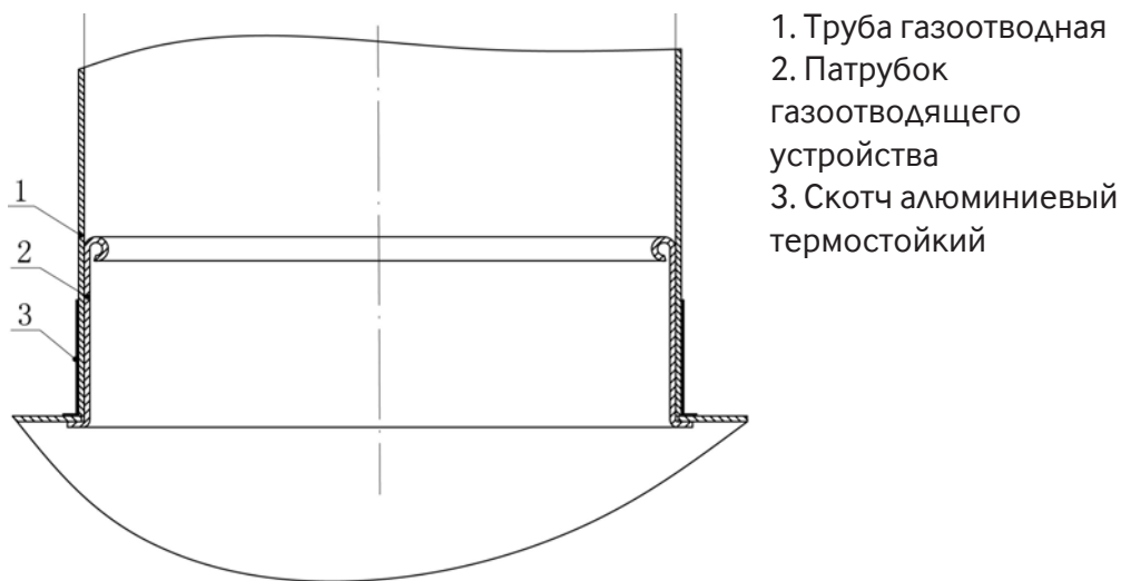
Рисунок 10. Схема подсоединения газоотводящей трубы
