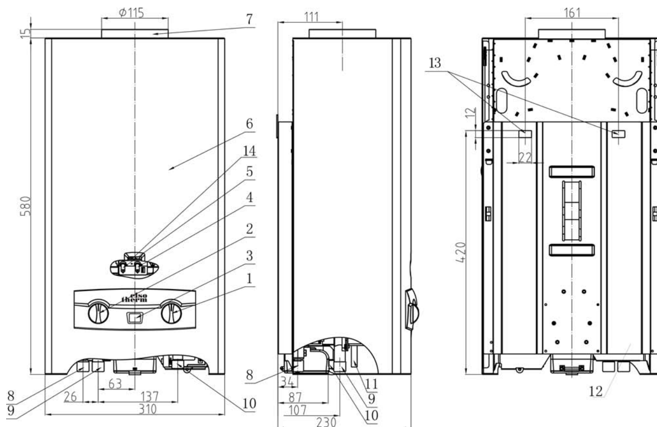
Рис.1 Внешний вид и присоединительные размеры аппарата
