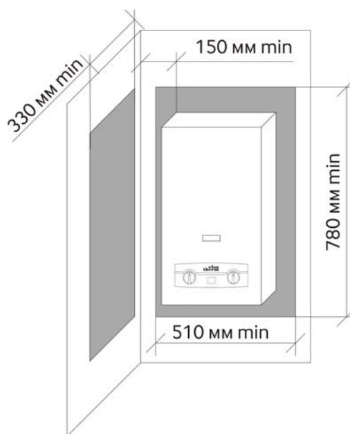
Рисунок 8. Установка аппарата на стене
