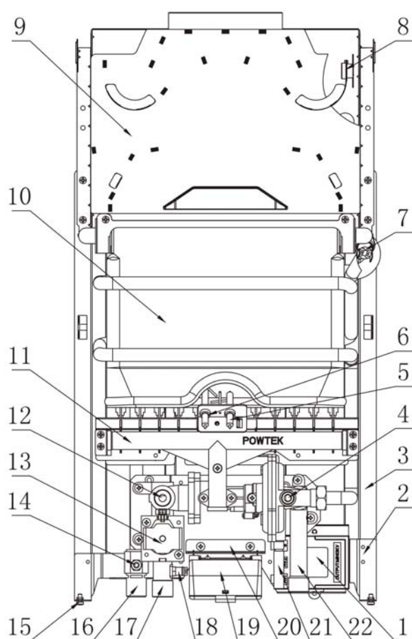
Рис. 2 Внутреннее устройство аппарата
